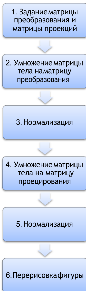
Рис. 10.4. Процесс визуализации трехмерного тела
