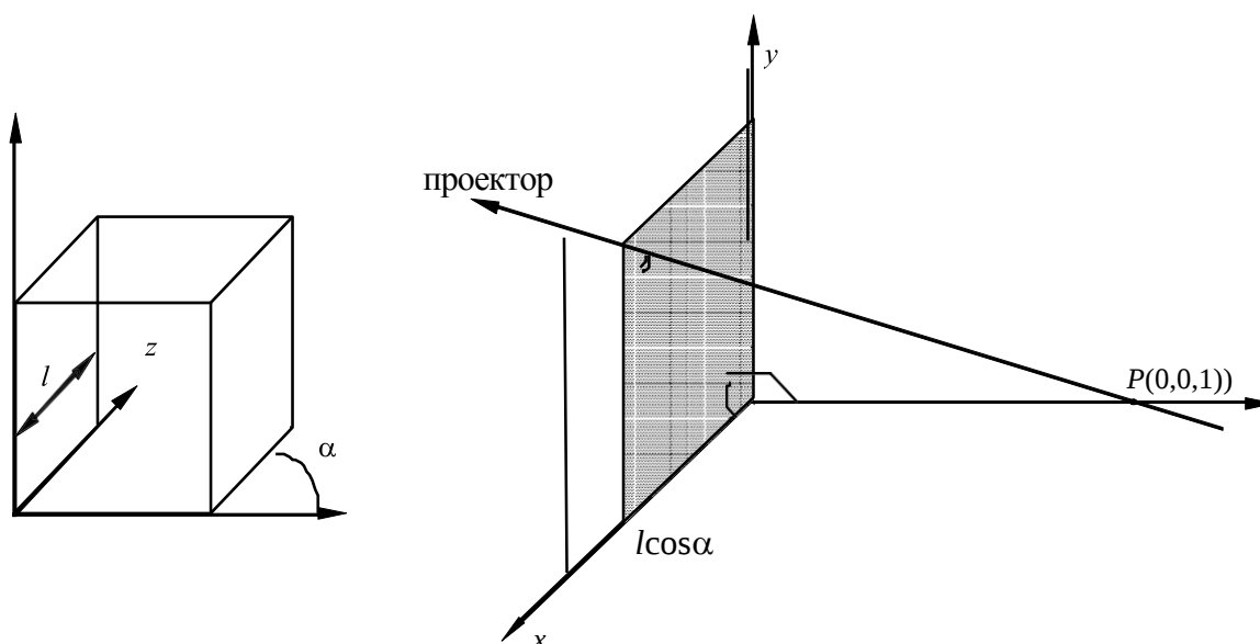
Рис. 10.3. Косоугольные проекции
