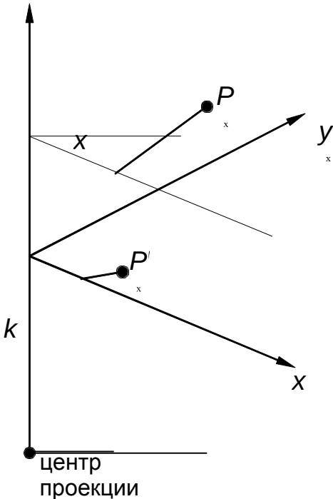
Рис. 10.2. Вычисление однотоочечной перспективы
